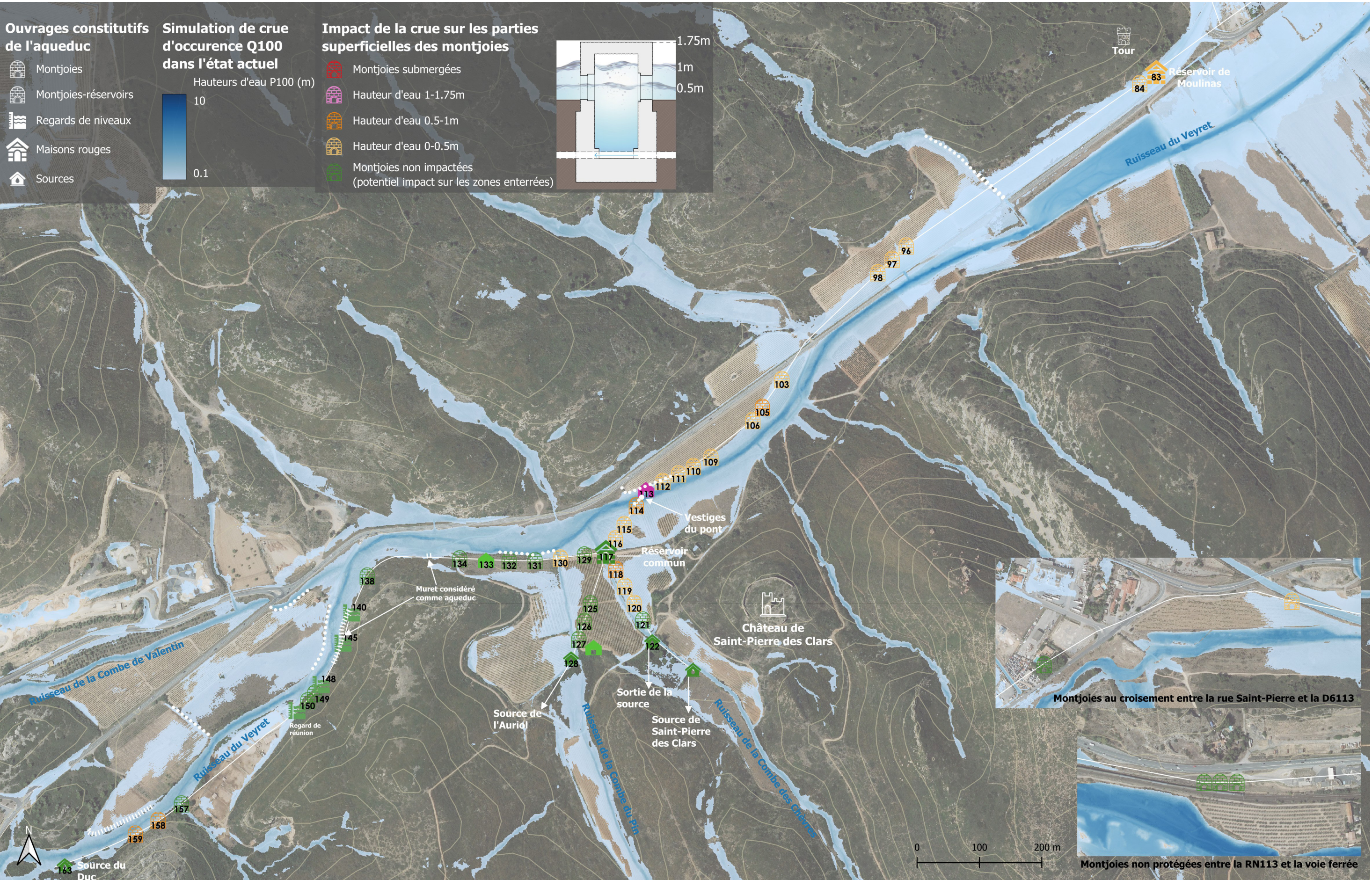
Carte de vulnérabilité de l'aqueduc des sources de Fontfroide - Etat actuel suivant la crue d'occurrence Q100
