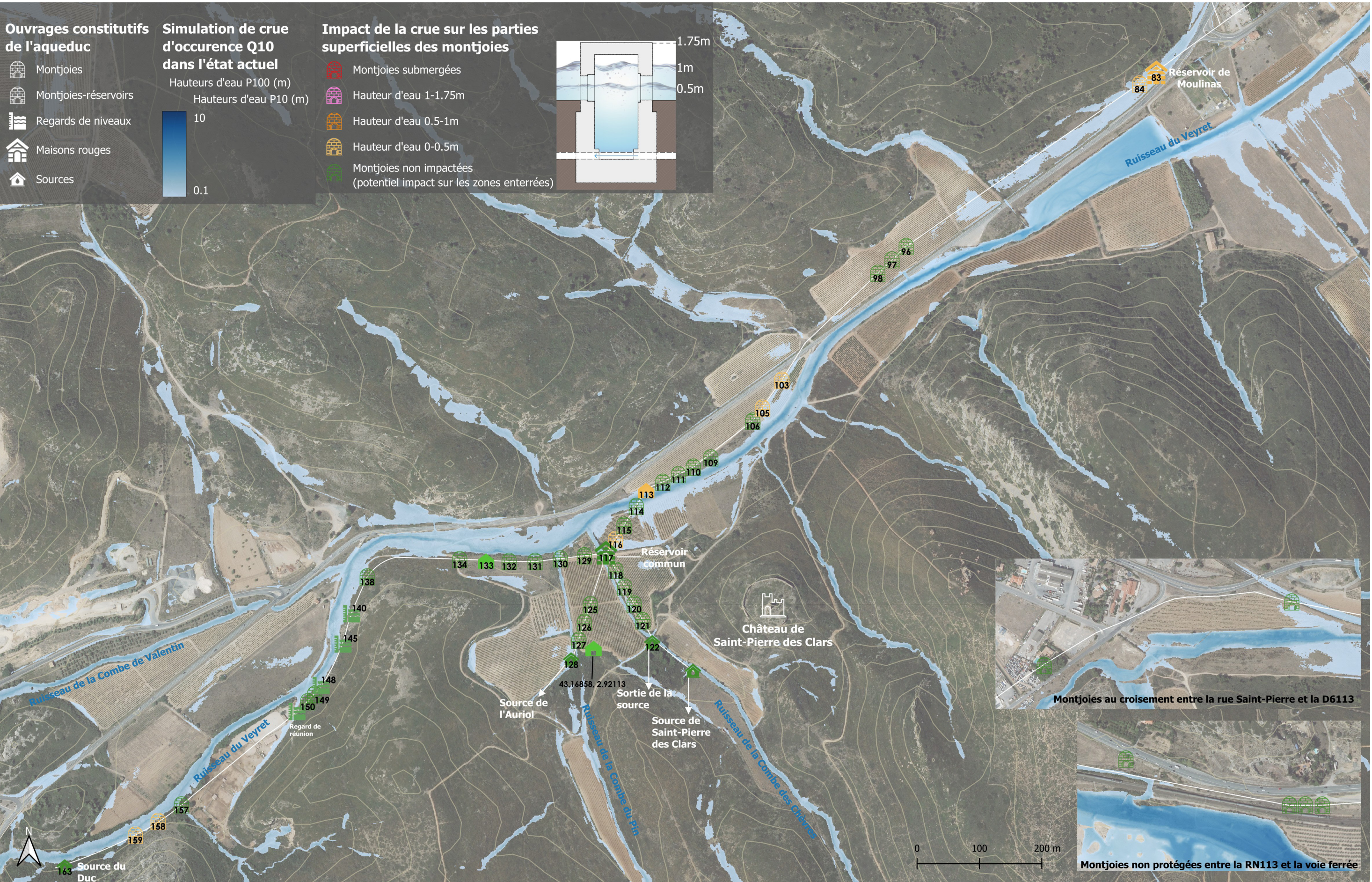
Carte de vulnérabilité de l'aqueduc des sources de Fontfroide - Etat actuel suivant la crue d'occurrence Q10
